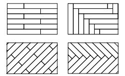
10x60 SUGGESTED LAYOUT EJEMPLO COLOCACIÓN 10x60 EXEMPLE DE POSE 10x60
